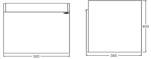
Plano acotado del Vanity:
